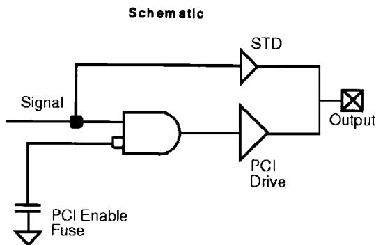
Figure 6• I/O Module
